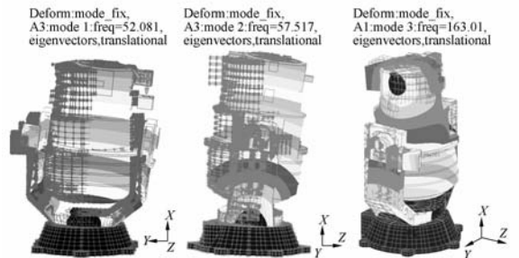
(a) Z 向基频振型 (b) Y 向基频振型 (c) X 向基频振型 (a) Nephogram of Z axis (b) Nephogram of Y axis (c) Nephogram of X axis
