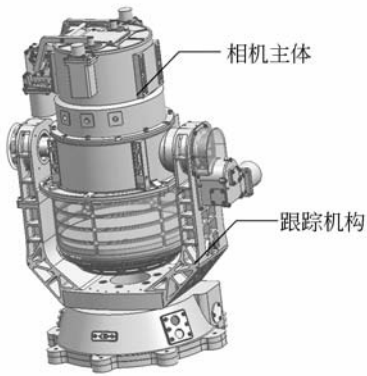
图 2 EUV 相机光机结构模型
