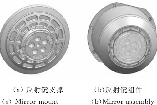
图 3 反射镜支撑及组件
